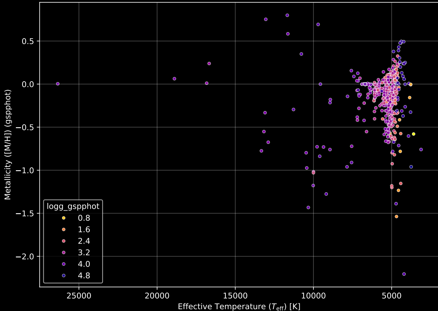
APOGEE DR17 Field: [210+00] Stellar Population Parameters (n= 514)
